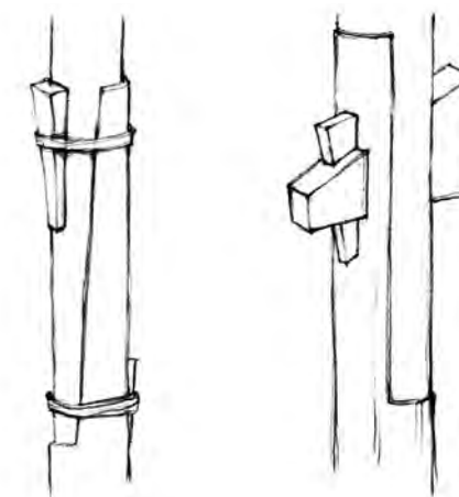
Рис. 15. Варианты сращивания осевого столба
