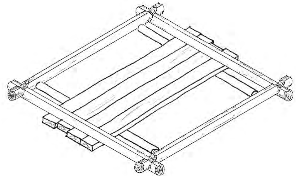
Рис. 2. Пол по бревнам-лагам, доски пола прижаты срубом
