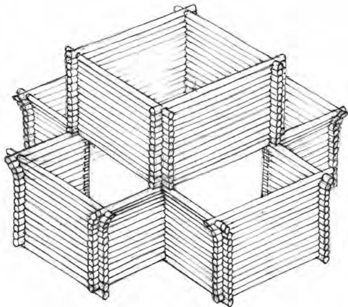
Рис. 17. Конструкция перехода от крещатого основания с повалами к широкому четверику
