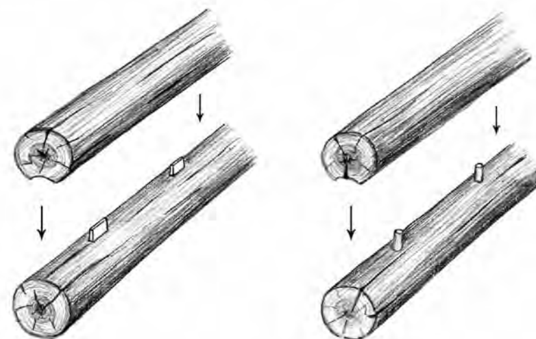
Рис. 6. Пластинчатые и стержневые нагеля
