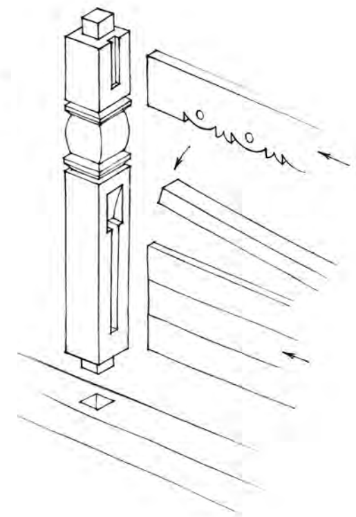
Рис. 5. Конструкция ограждения площадки крыльца или галереи
