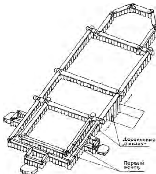
Основание (фундаменты) из деревянных студьев и первый (окладной) венец Никольской ц. в Высоком Острове. XVIII в. Реконструкция.
