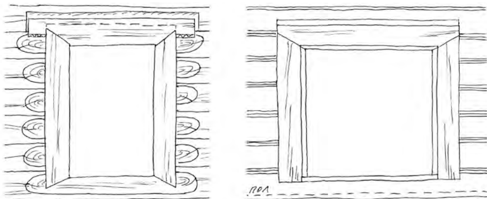
Рис. 9. Типы дверных проемов XVII–XVIII веков. Слева — дверь со стороны паперты, придела. Боковые косяки врублены в порог «косо». Справа — широкая дверь со стороны церкви. Боковые косяки врублены в порог прямо
