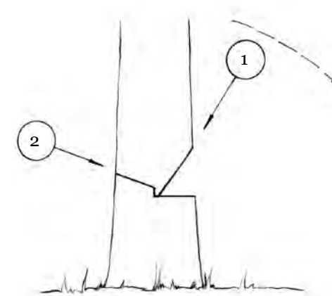
Рис. 3. Схема валки дерева при помощи топора
