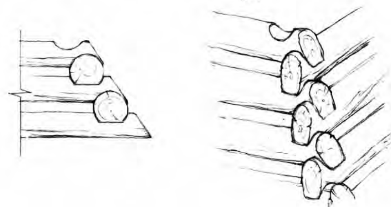
Рис. 10. Рубленое четырехскатное покрытие
