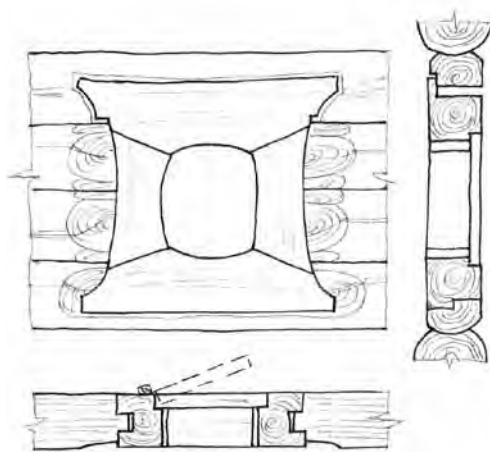
Рис. 7. Окно в алтаре церкви Рождества Богородицы (1531 год) из с. Передки. Вид на фасаде, план, разрез (по Л. Е. Красноречьеву)
