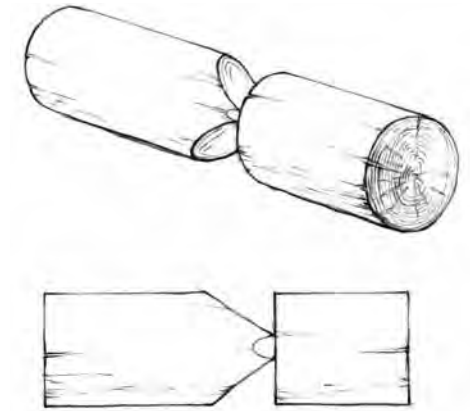
Рис. 8. Перерубка бревна поперек волокон
