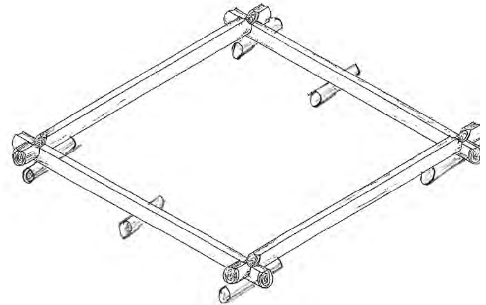
Рис. 2. Сруб на угловых и промежуточных подкладках
