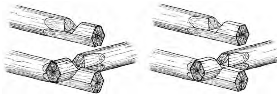
Рис. 11. Модификации соединения «в шведский угол». Разная припазовка
