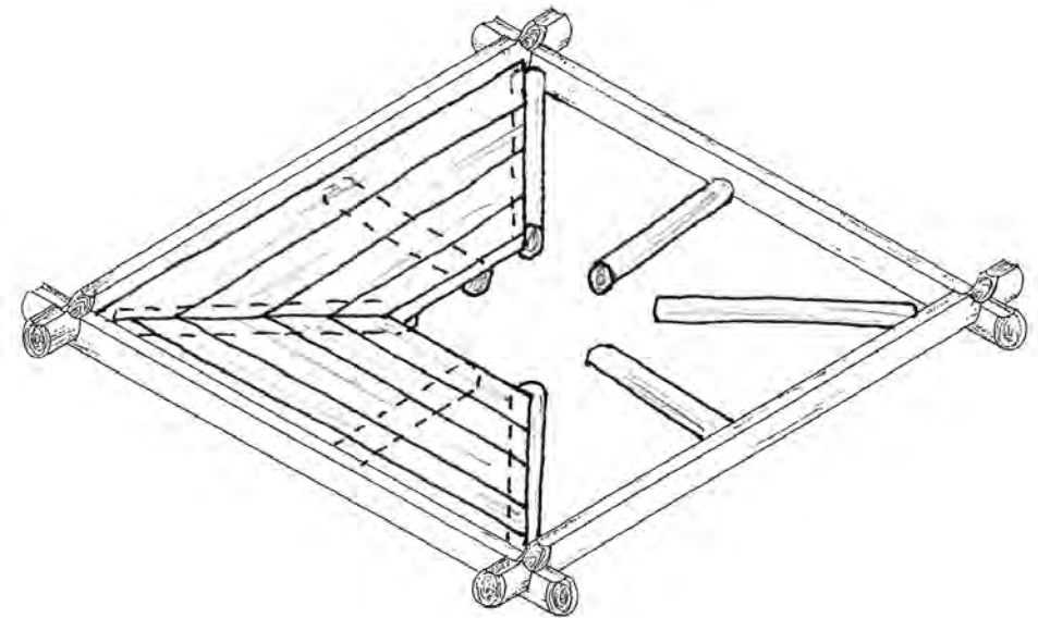
Рис. 3. Полы, уложенные параллельно каждой стене
