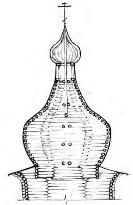
Рис. 13. Рубленая конструкция восьмигранной пучины
