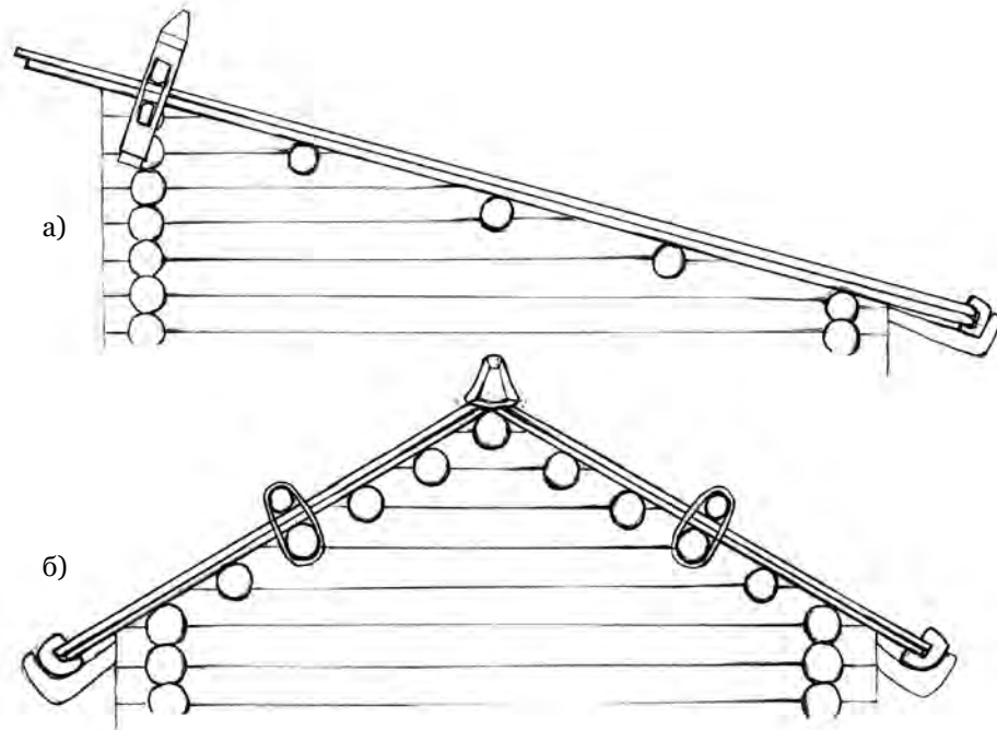
Рис. 14. Конструкции безгвоздевых самцово-слеговых кровель: а) односкатной с гнетами и «чиби»; б) двухскатной с гнетами, перевязанными лыком
