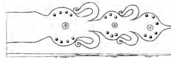
Рис. 21. Фрагмент «жиковины» из церкви Успения. Обмер А. В. Ополовникова, 1958 год
