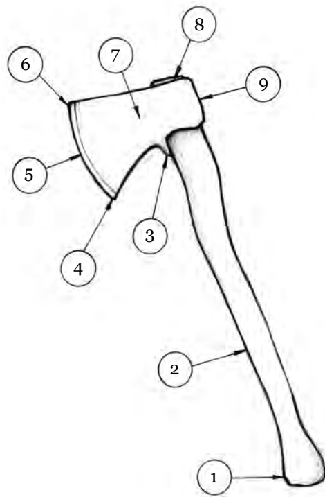
Рис. 3. Названия элементов топора: 1 — хвост, 2 — хват, 3 — бородка, 4 — пятка, 5 — лезвие, 6 — носок, 7 — боек, 8 — проушина, 9 — обух
