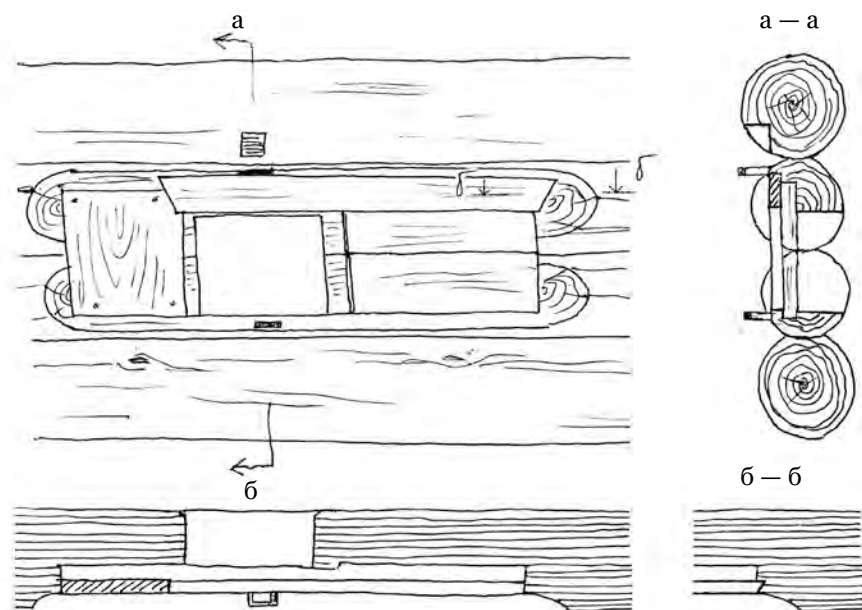
Рис. 3. Волоковое окон в южном приделе церкви Рождества Богородицы из с. Перёдки. Общий вид в интерьере, план, разрез до реставрации; б — б сечение по концу планки
