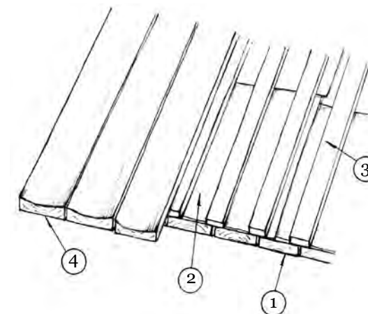
Рис. 3. Кровля в два теса с прокладкой скалы (бересты) и драни: 1 — нижний слой теса; 2 — скала; 3 — дрань; 4 — верхний слой теса
