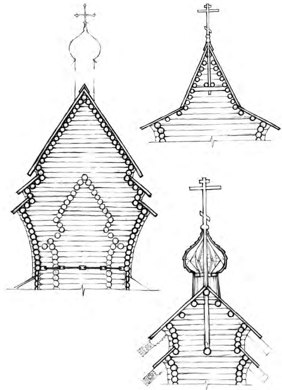
Рис. 3. Варианты сложных коньковых покрытий. Клинчатая с полницами и каскадная крыша
