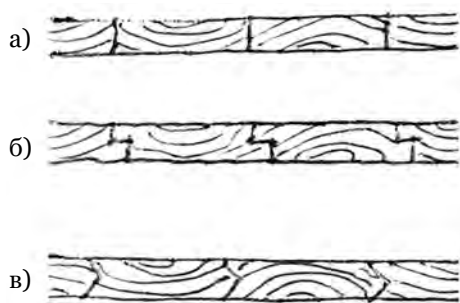
Рис. 8. Способы однорядного соединения тесин: а) ровными краями, б) «в четверть», в) «гребнем в паз»
