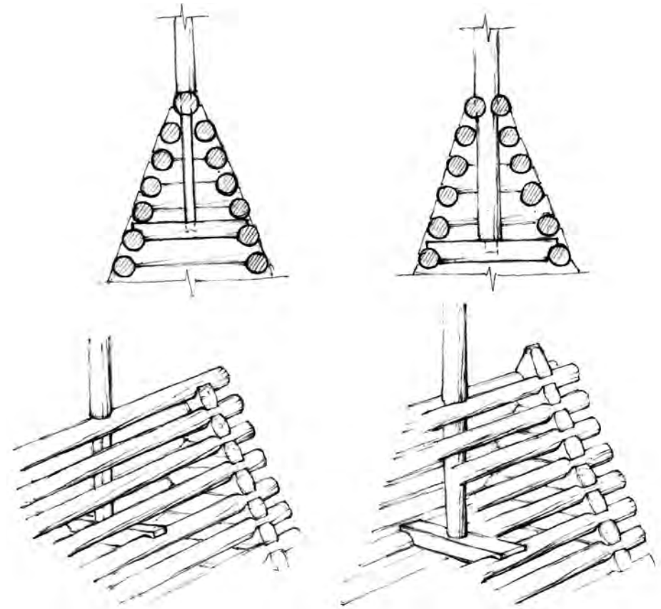
Рис. 6. Варианты установки столба главы или креста на островерхое двухскатное покрытие
