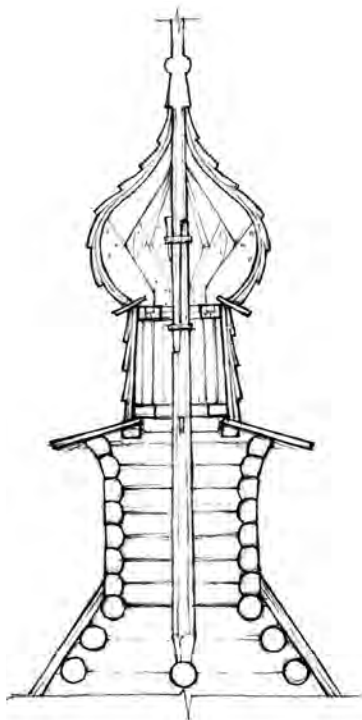
Рис. 7. Установка на двухскатное покрытие яруса-постаменты под главу
