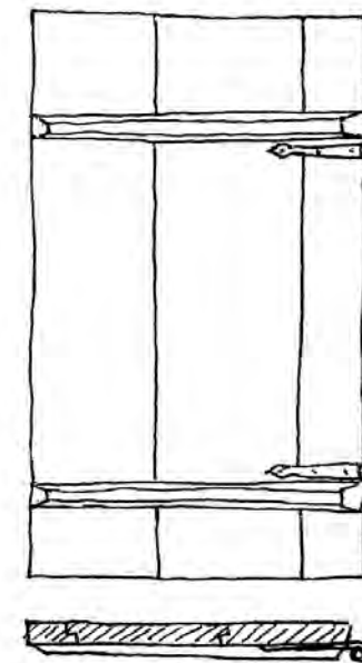
Рис. 18. Типичное дверное полотно на металлических петлях
