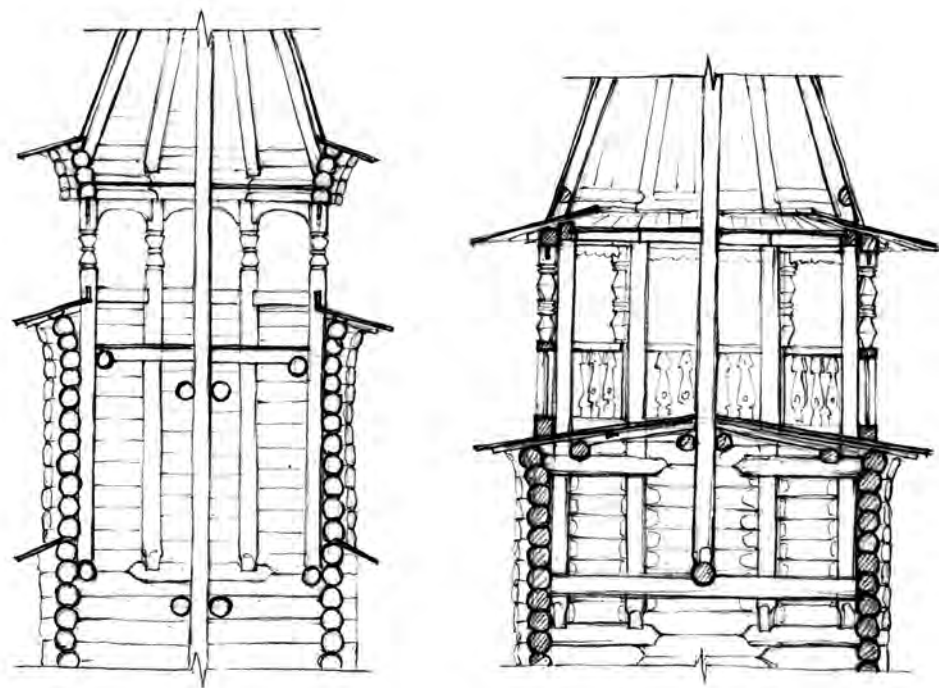
Рис. 18. Конструкции каркасных завершений колоколен
