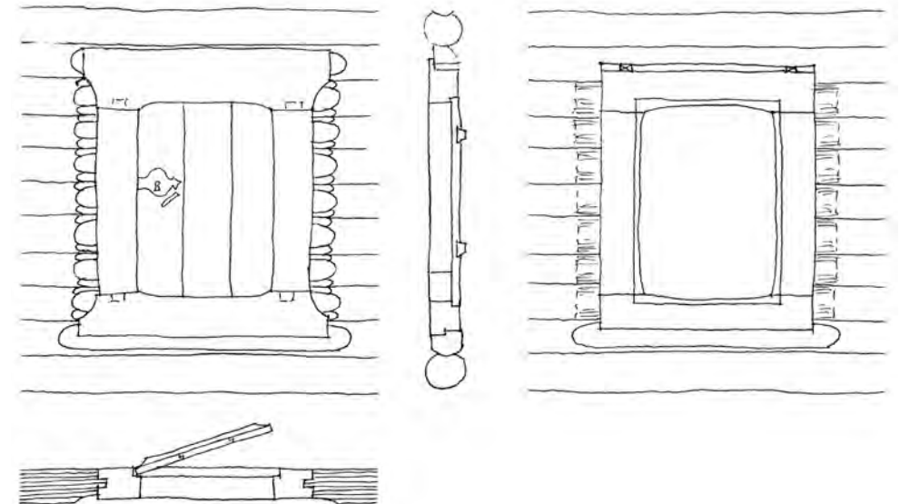
Рис. 4. Дверь в церкви Рождества Богородицы из с. Перёдки. Вид на фасаде, разрез, вид в интерьере, план (по Л. Е. Красноречеву)
