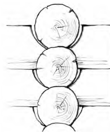
Рис. 10. Щели в угловых соединениях после усушки бревен
