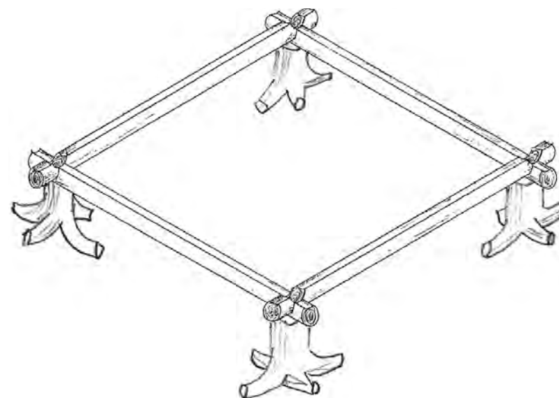
Рис. 11. Сруб «на куриных ногах»
