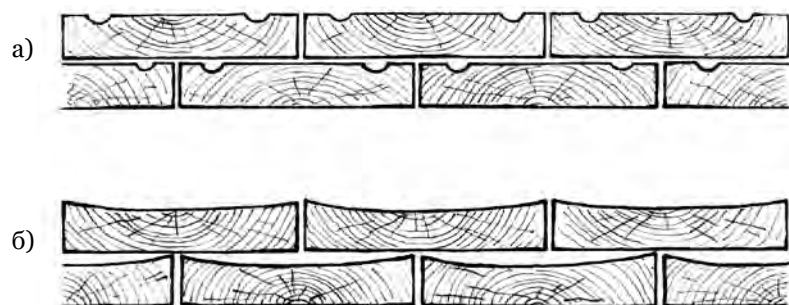
Рис. 10. Схема укладки теса: а) дороженого; б) ложенного
