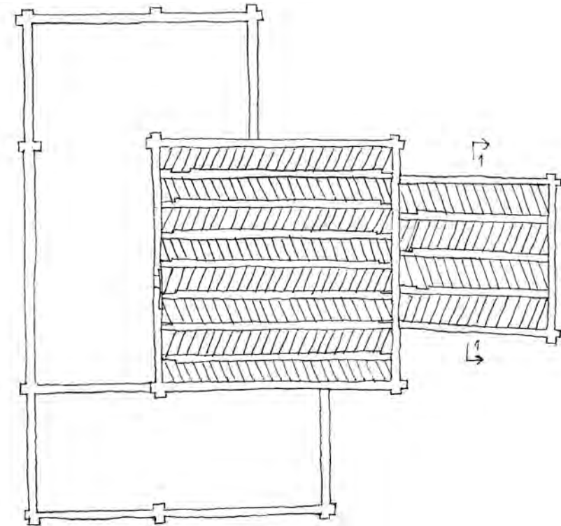
Рис. 11. Потолок в церкви Успения из с. Курицко
