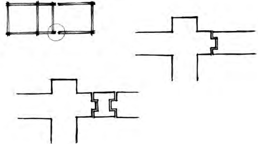
Рис. 5. Сращивание стен дома и хозяйственной части
