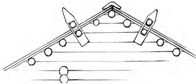
Рис. 13. Конструкция безгвоздевой самцово-слеговой кровли с гнетами, «чиби» и охлупнем
