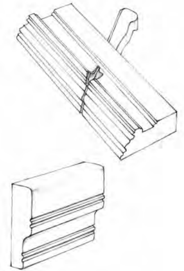
Рис. 46. Калевочник. Фрагмент подзора с калевками
