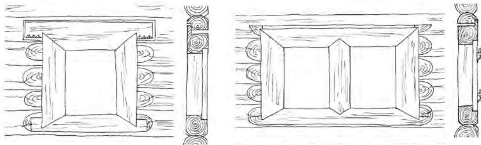
Рис. 9. Пример раннего трехкосящатого окна с имитацией нижнего косяка. Вид на фасаде, разрез
