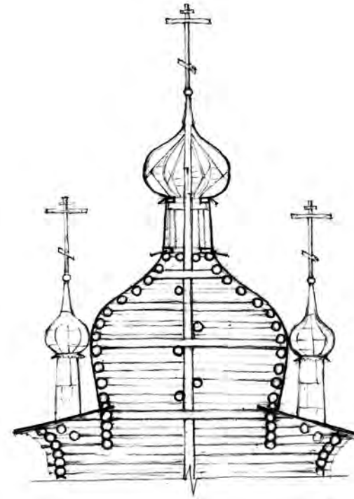
Рис. 12. Рубленая конструкция кубоватого покрытия
