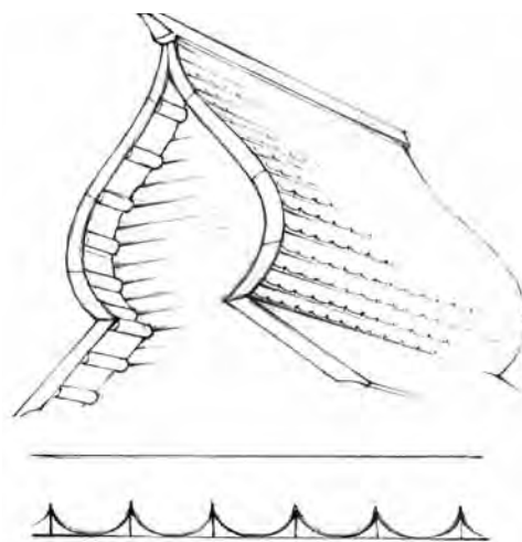
Рис. 20. Бочка покрытая, горизонтальным тесом с полукруглыми. Фрагмент тесовой доски
