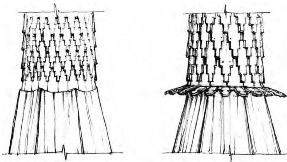
Рис. 12. Варианты переходов от восьмигранного шатра к круглой шее
