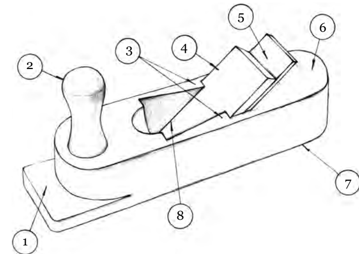
Рис. 42. Названия элементов рубанка: 1 — нос; 2 — рукоятка; 3 — заплечики; 4 — клин; 5 — нож; 6 — задняя «бабка»; 7 — колодка; 8 — зев
