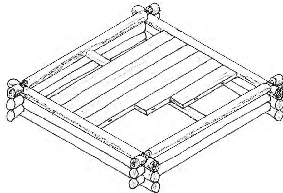
Рис. 8. Половицы прижаты срубом
