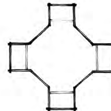
Рис. 8. Восьмигранный в плане основной сруб с четырьмя прирубами. Внутри прирубов — связи
