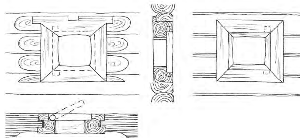
Рис. 6. Окно в алтаре церкви Ризоположения (1485 год). Общие виды, план, разрез (по А. В. Попову)
