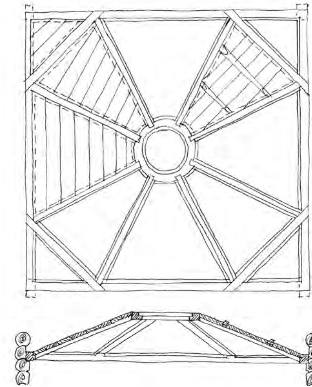
Рис. 18. Схема каркасных «небес» на 8 граней с примерами различных заполнений граней. План, разрез
