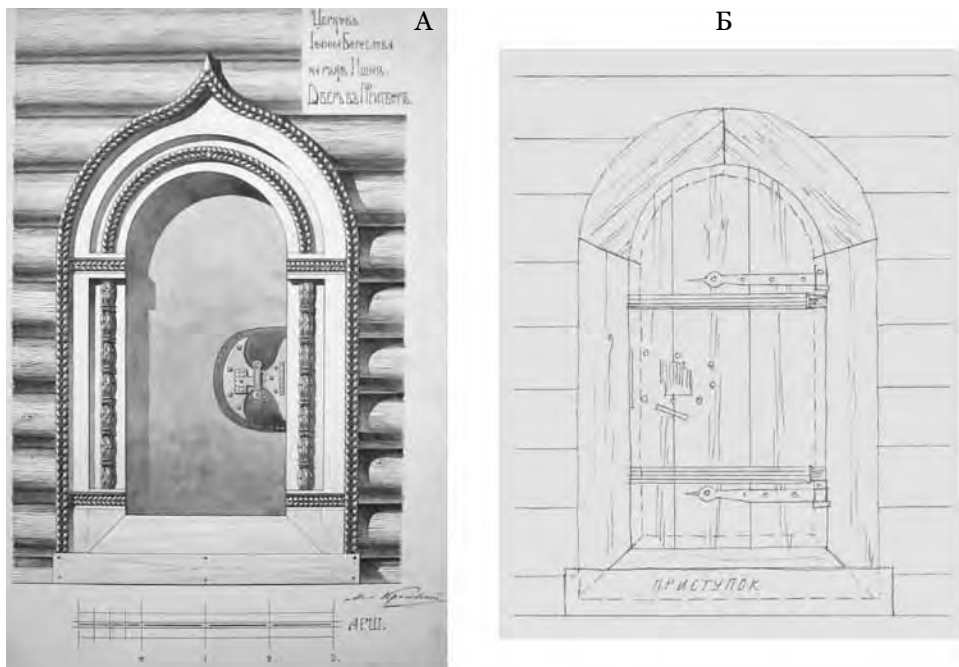
Рис. 8. Дверь в церкви Иоанна Богослова на р. Ишня. А — вид со стороны паперты (чертеж М. Красовского, 1906 год), Б — вид со стороны трапезной
