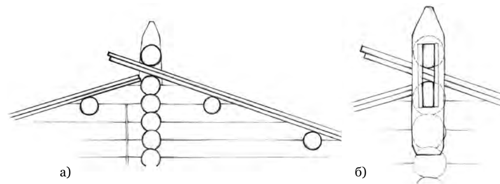
Рис. 12. Конструкция безвоздевой самцово-слеговой кровли с гнетами и «чиби»: а) фрагмент разреза; б) фрагмент фасада
