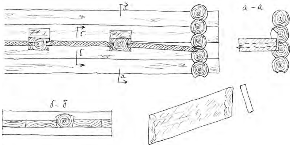
Рис. 10. Фрагменты, узлы и детали потолка в церкви Рождества Богородицы из с. Перёдки
