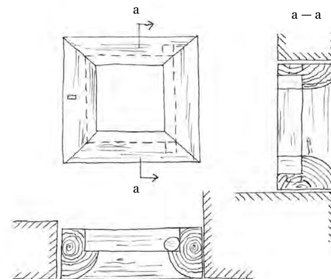
Рис. 5. Обрамление ниши в церкви Спаса на Нередице. Общий вид, план, разрез
