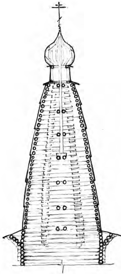
Рис. 11. Рубленая конструкция шатра
