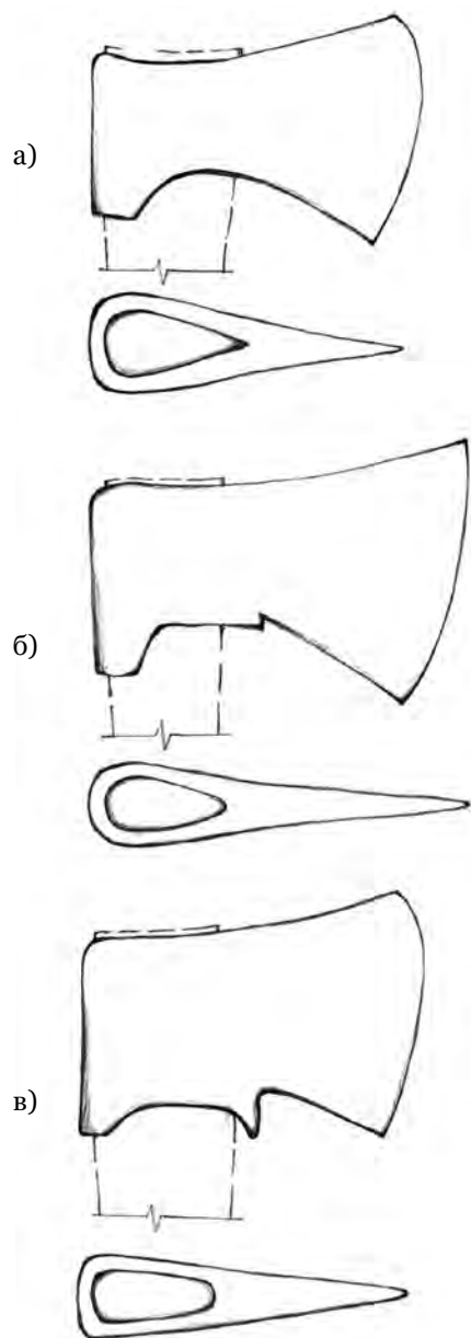
Рис. 5. Топоры, найденные на Мангазейском городище: а) I группа — топоры конца XVI; б) II группа — топоры конца XVI — первой половины XVII веков; в) III группа — топоры XVII века
