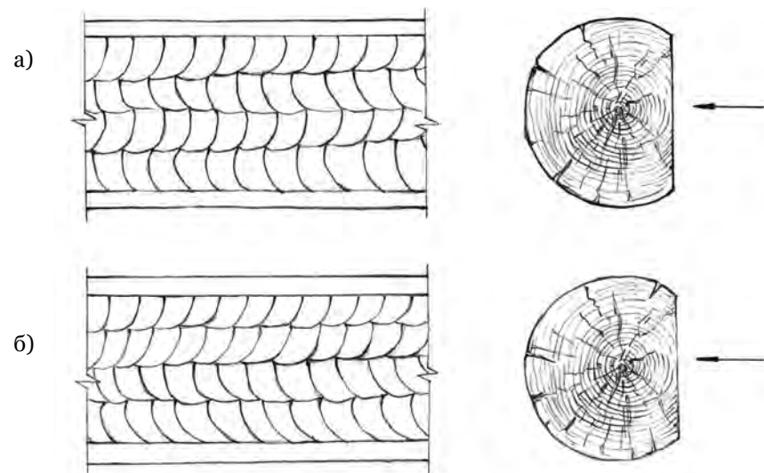
Рис. 10. Схемы направления тески: а) при прямослойной древесине; б) при косослойной древесине (по материалам А. В. Попова)
