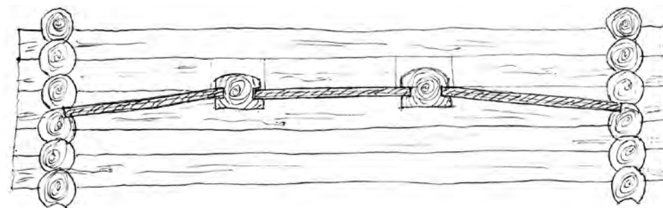
Рис. 6. Потолок с двумя балками «двутаврового» сечения
