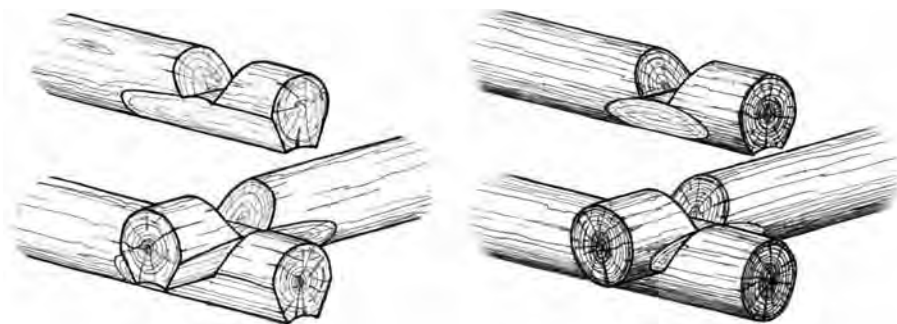
Рис. 9. Угловое соединение с трапециевидной формой чаши
