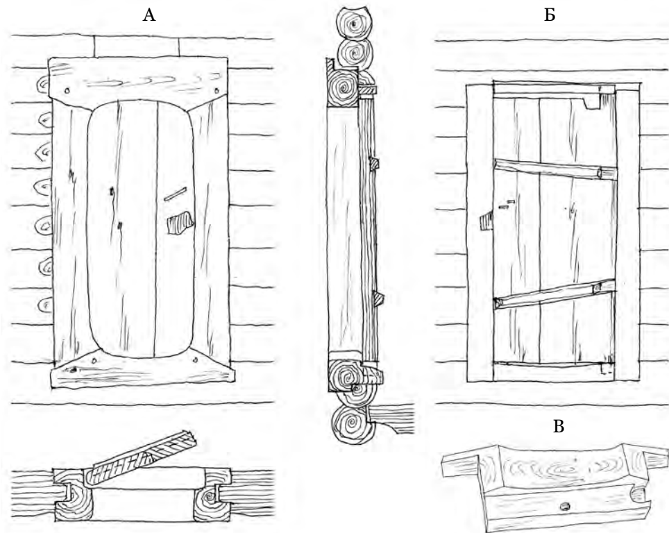
Рис. 3. Южные двери церкви Воскрешения Лазаря. А — вид на фасаде, Б — вид в интерьере, В — порожняя колода; разрез, план (по А. В. Ополовникову)
