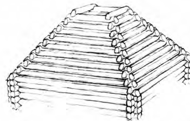
Рис. 9. Крещатое восьмискатное покрытие и крещатая «бочка»
