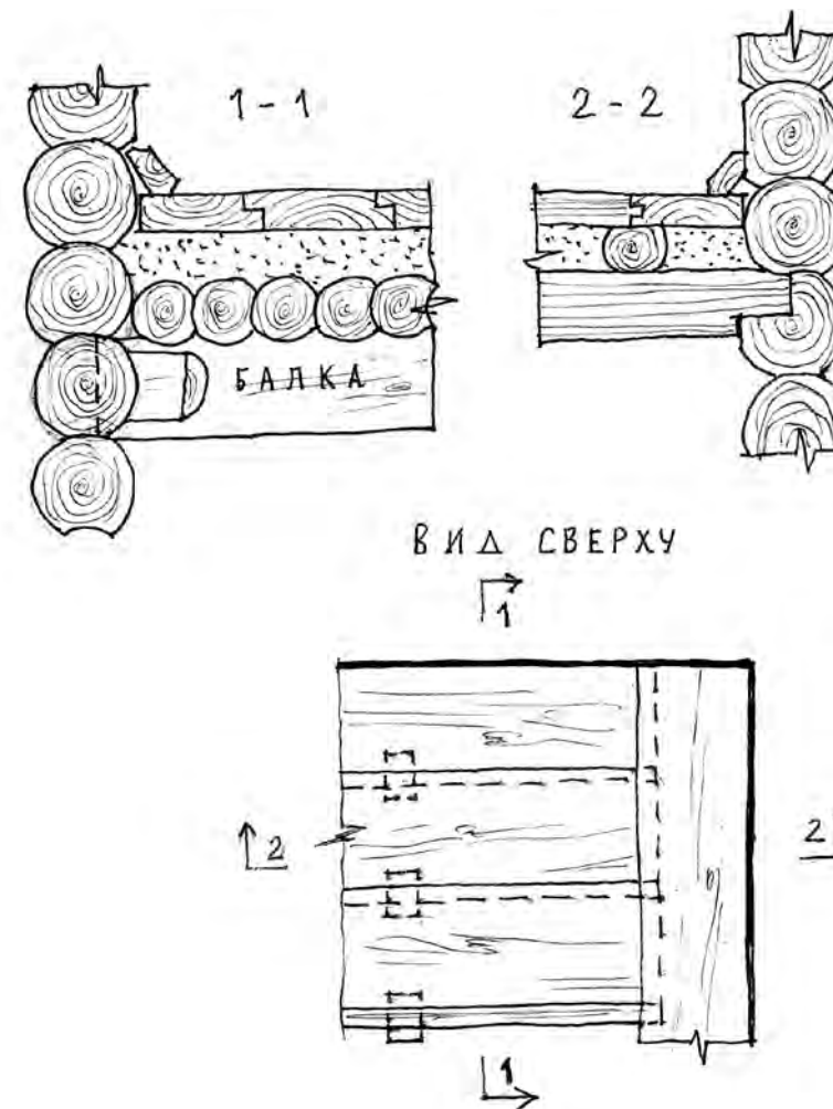
Рис. 10. Узлы двойных полов. Фрагмент фризového пола
