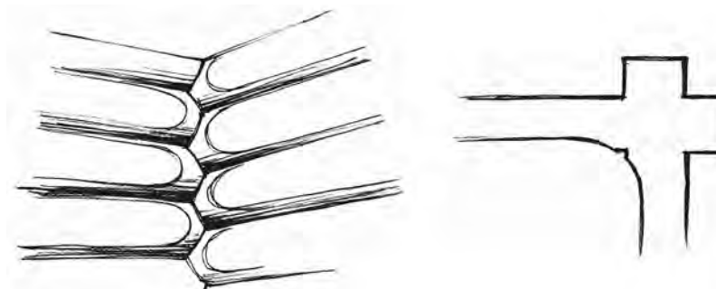
Рис. 24. Отеска стен «в круглый угол»
