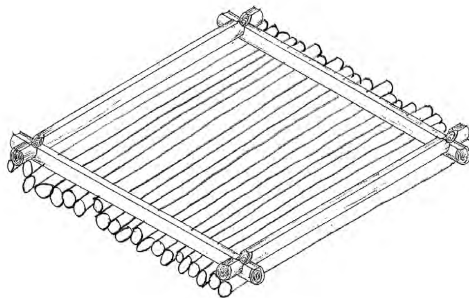
Рис. 5. Сруб на сплошной бревенчатой вымостке
