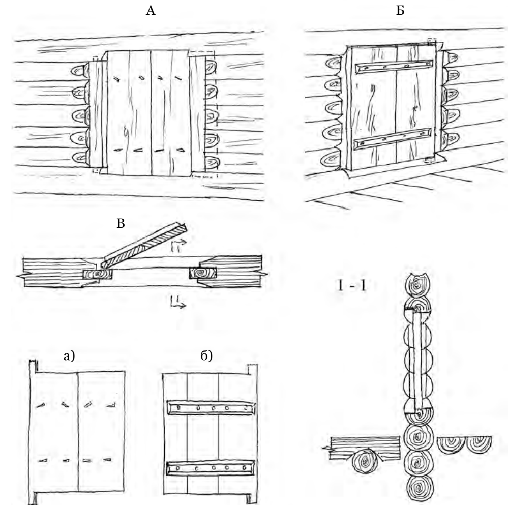
Рис. 1. Устройство дверных проемов в X–XIII веков:
