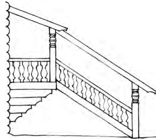
Рис. 2. Односходное крыльцо на консолях
