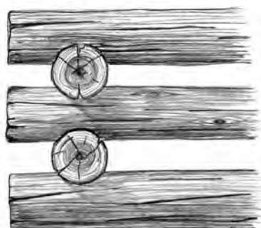
Рис. 23. Рубка «в режь»
