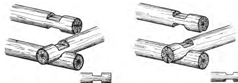
Рис. 12. Угловое соединение «в охряпку»
