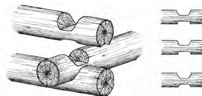
Рис. 16. Угловая врубка «в полуторную чашу». Варианты форм чаш
