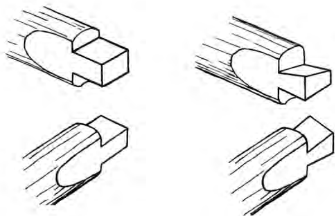
Рис. 18. Соединения «в лапу»
