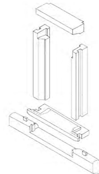
Рис. 13. Коробка оконного проема (конец XIX — начало XX веков) в разобранном виде. Вид со стороны интерьера. Снизу — вверх: нижнее бревно с шипами для колод и коксами, подоконник — «подушка», боковые брусья, вершник
