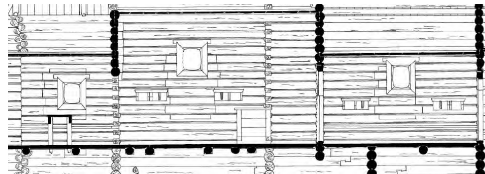
Рис. 27. Никольская церковь. Фрагмент разреза с видом на юг. Чертеж Л. Е. Красноречьева
