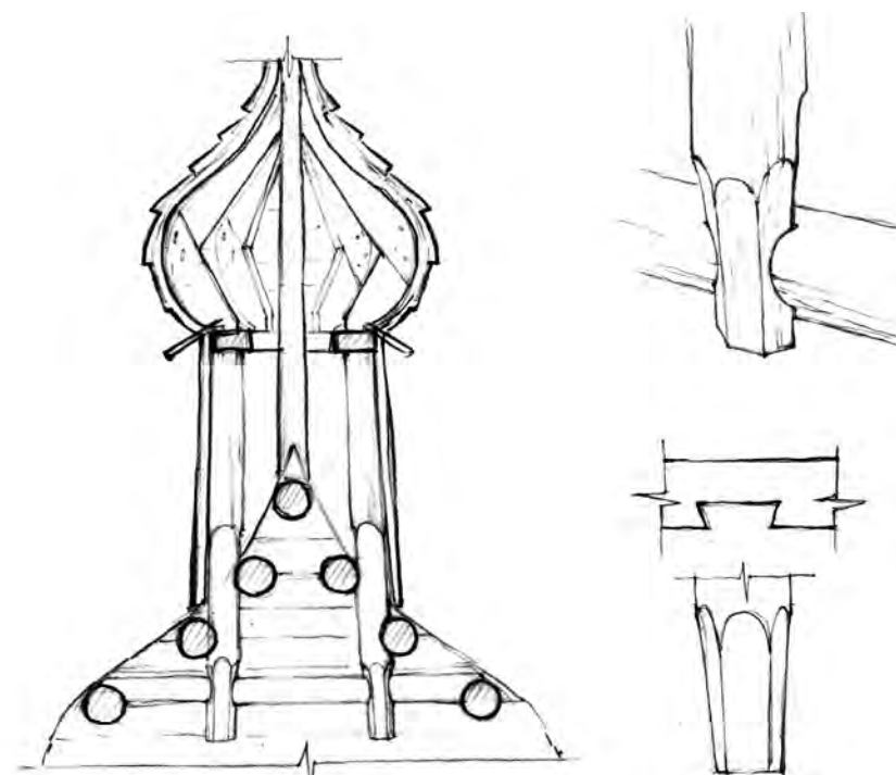
Рис. 13. Конструкция главы с шей на четырех стойках
