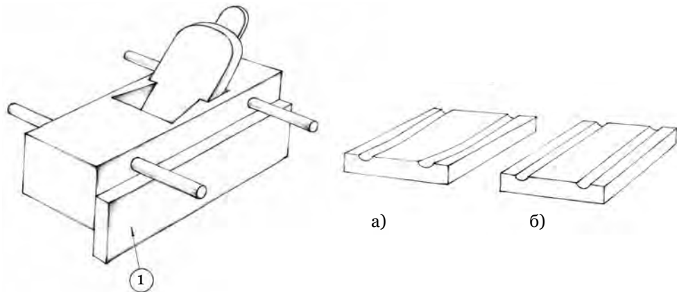
Рис. 45. Дорожник. 1 – упор. Дорожки на тесе выполнены дорожником: а) без упора; б) с упором
